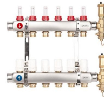
BASE Set distribuitor inox cu diblmetru 4 căi 1" 6085620 5 căi 1" 6085630 6 căi 1" 6085640 8 căi 1" 6085660
