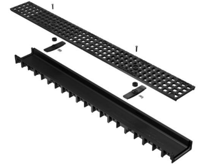
Rigola 100H30 + gratar fonta retea trafic 12.5 tone+Sistem de fixare 100x120x54,5
